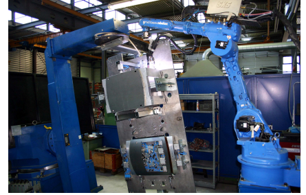
Roboter Motoman HP-20 mit H-Tisch
